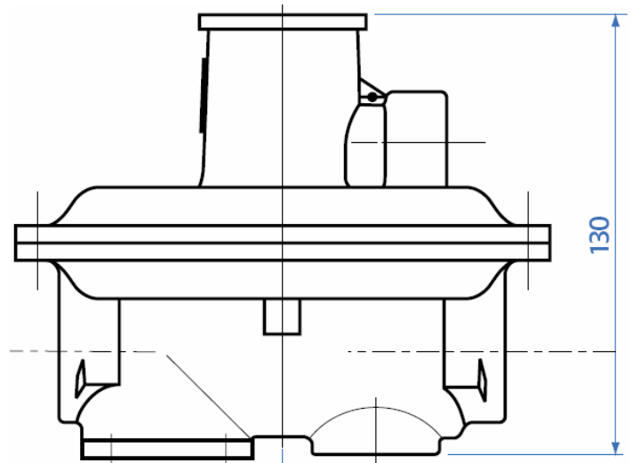
Регулятор серии RB 1210 (без ПЗК) Вес: 1,0 кг.
